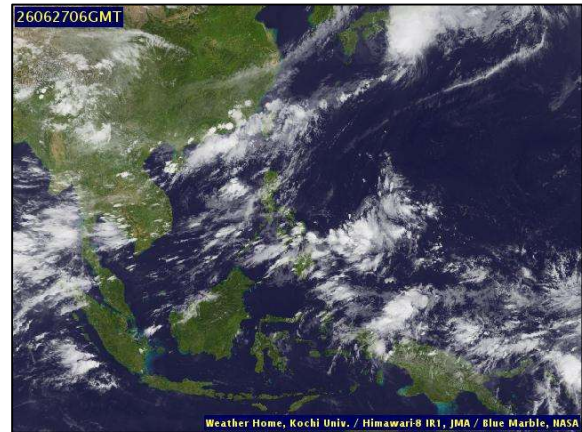
ภาพถ่ายดาวเทียม วันที่ ๒๗ มิ.ย. ๒๕๖๙ เวลา ๑๓.๐๐ น.
