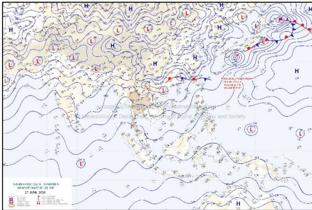
แผนที่อากาศ วันที่ ๒๗ มิ.ย. ๒๕๖๙ เวลา ๑๕.๐๐ น.
